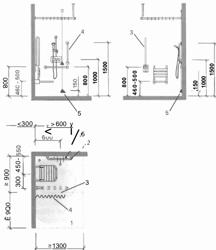
Obrázek 34- Bezbariérový sprchový kout
