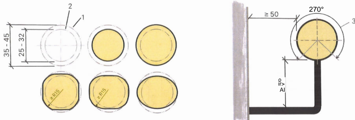
Obrázek 18 - Zábradelní madlo - umístění a tvarové řešení
