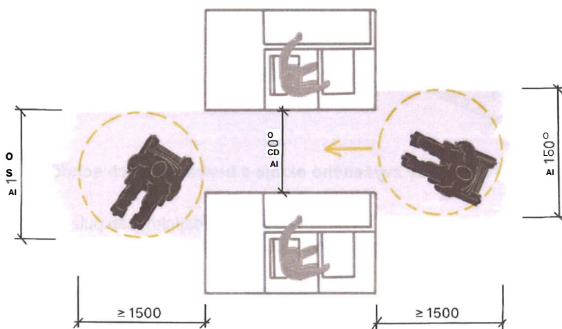
Obrázek 42 - Průchodí a manipulační prostor u pokladních pásů
