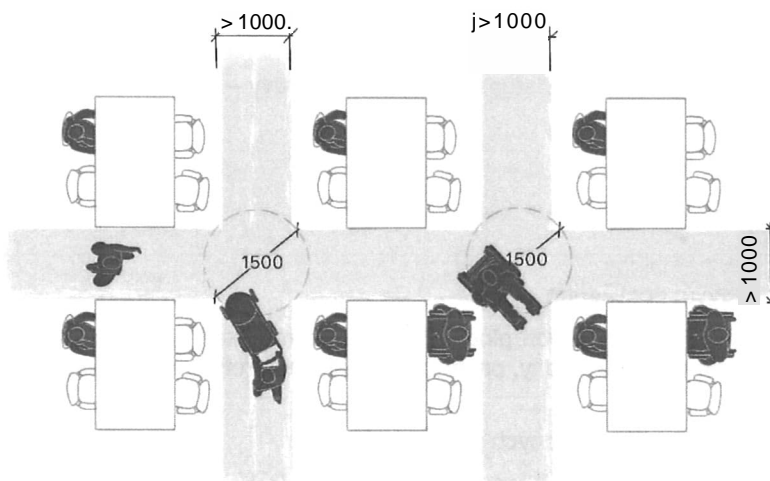
Obrázek 43 - Příklad s parametry průchozích a manipulačních prostorů v restauračním provozu
