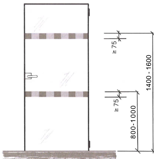
Obrázek 10 - Parametry minimálního kontrastního značení prosklených ploch
