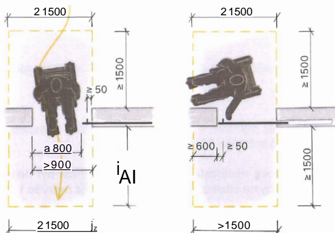
Obrázek 11 - Manipulační prostor u posuvných dveří
