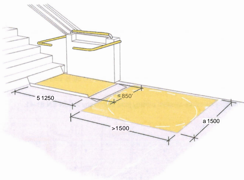
Obrázek 24 - Manipulační prostor u šikmé zvedací plošiny v poloze přímé, otočené o 180^\circ a 90^\circ
