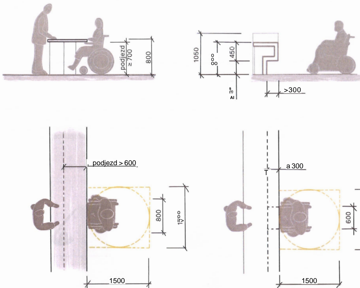
Obrázek 2 - Plný podjezd a částečný podjezd vozíku
