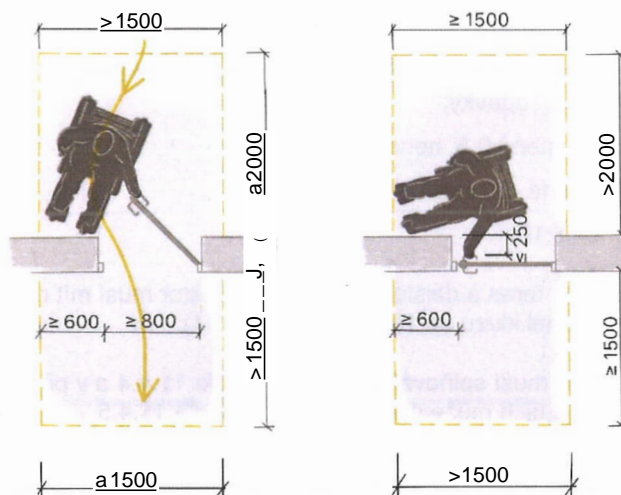
Obrázek 12 - Manipulační prostor u otevíracích dveří
