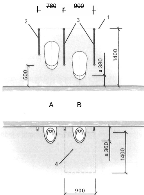
Obrázek 33 - PISOÁRY pro osoby s omezenou schopností pohybu
