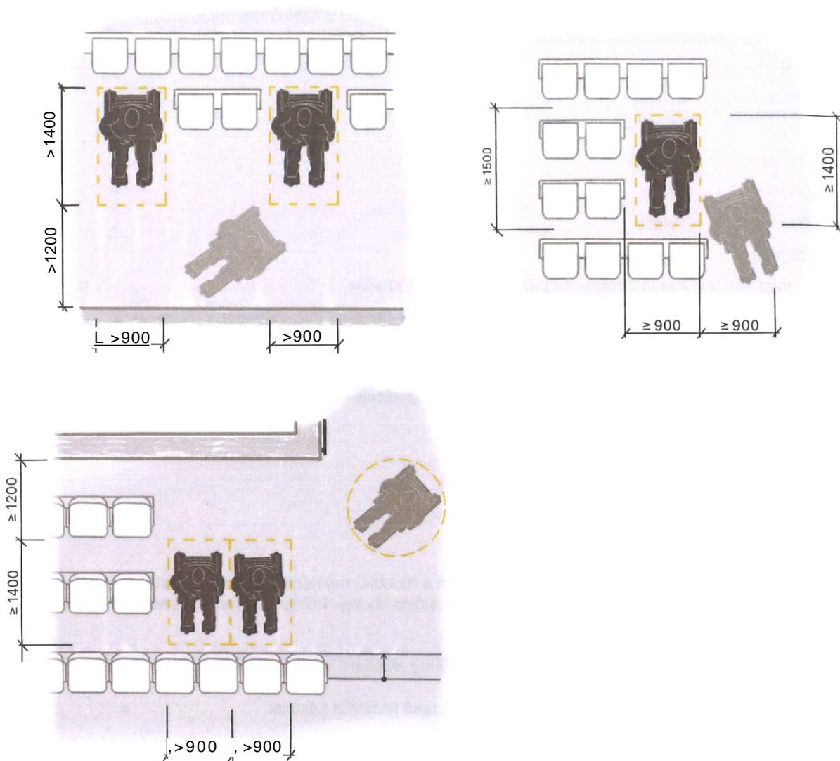
Obrázek 38 - Příklady umístění a parametry místa pro vozík v hledišti
