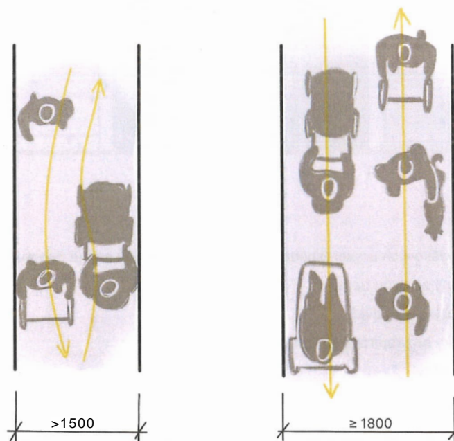
Obrázek 8 - Minimální průchodná šířka komunikačních prostor - chodby
